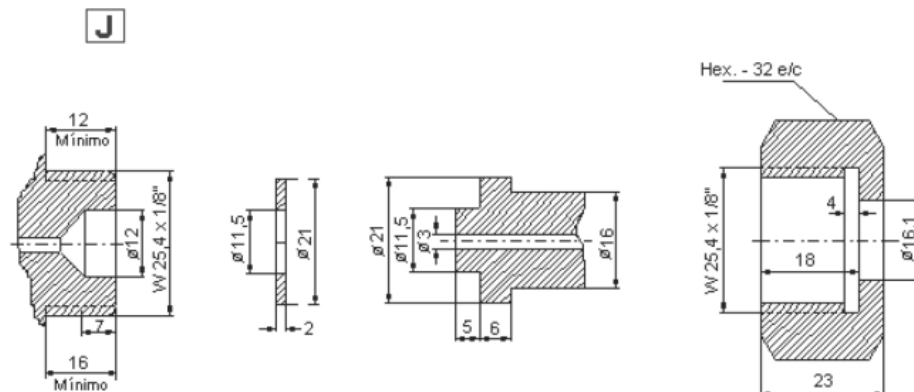
ACOPLAMIENTO W 25,4 - 8 Hilos/Pulgada (DERECHA) TIPO CORROSIVO Y TOXICO
