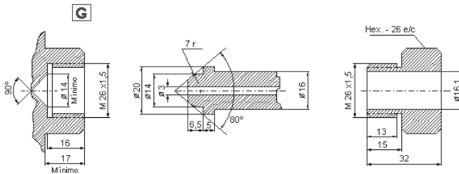
ACOPLAMIENTO M 26 x 1,5 METRICO (DERECHAS) TIPO COMBURENTES
