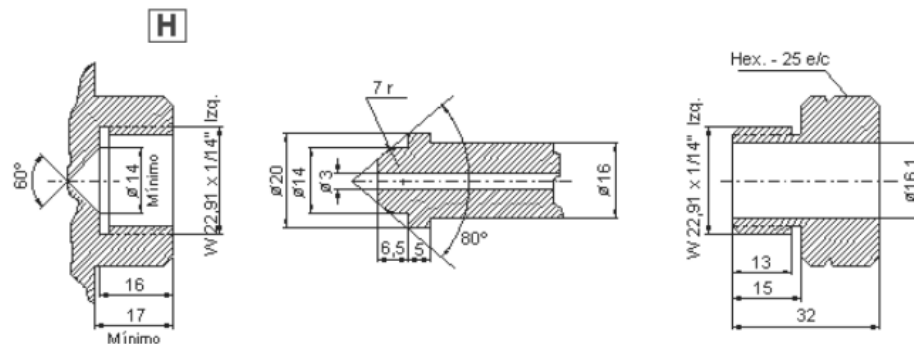
ACOPLAMIENTO W 22,91 - 14 Hilos/Pulgada (IZQUIERDAS) TIPO ACETILENO
